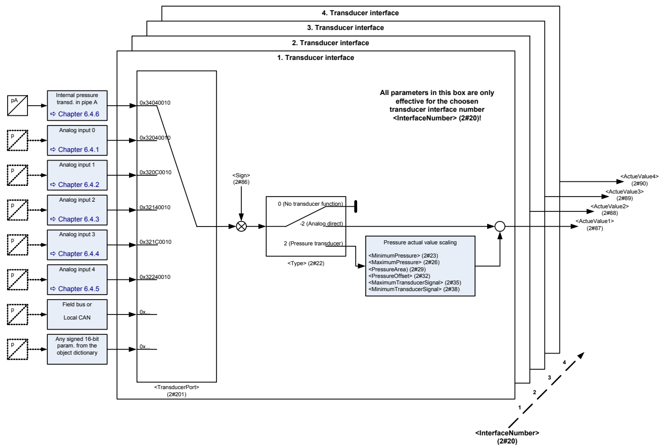
Figure 20: Actual value path
