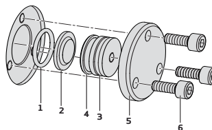
Abb.: Darstellung des Aufbaus
