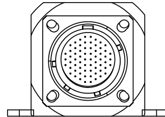
J1 D38999/20xF35PN
